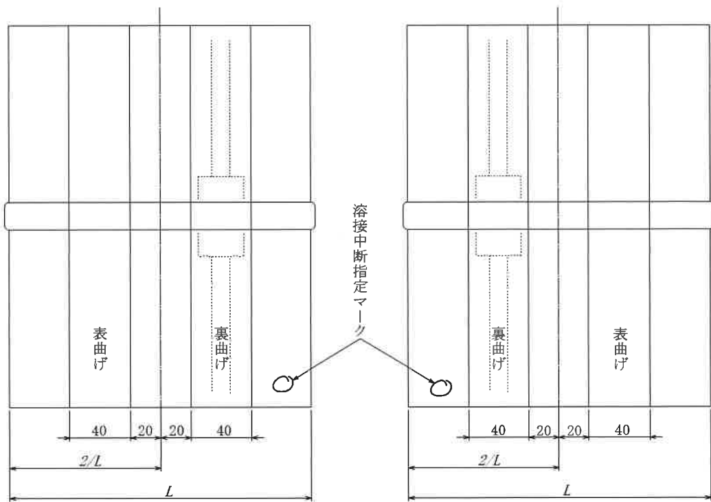
(A図: 溶接中断位置が右側の場合)
