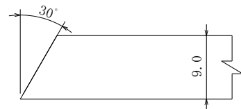
開先：べベル角度30°
