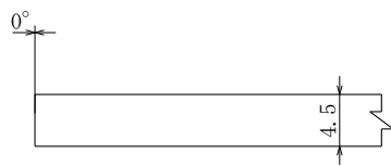
開先：I形
