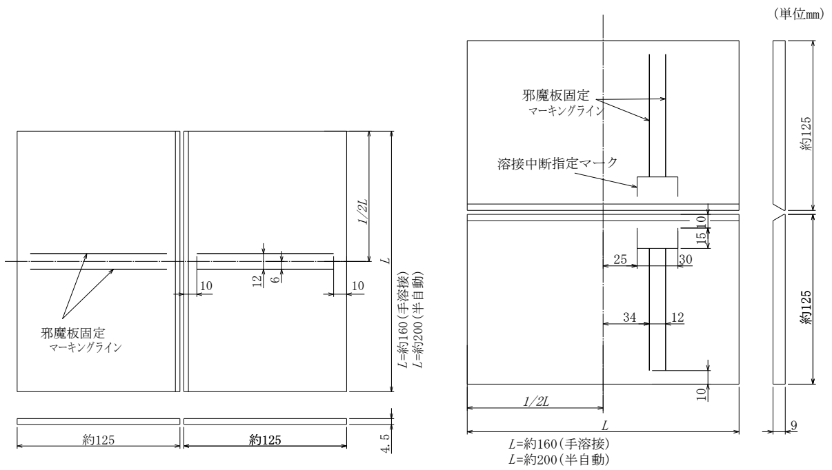
薄板競技材
